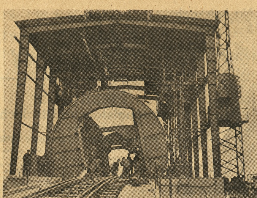
W szczecińskim porcie w dniu 7. 11. 51 w 34 rocznicę Rewolucji Październikowej na 5 dni przed terminem zostały uruchomione dwie wyrotnice wagonowe oraz urządzenie taśmowe do przeladunku węgla z wagonów kolejowych na statki. Urządzenie taśmowe przeladunku węgla wszystkich sortymentów od młodu do kęsów, o wadze do 130 kg włącznie. — Na zdjęciu: Obracający się węgla z wagonów, znajdujących się w wyrotnicy do zbiornika
