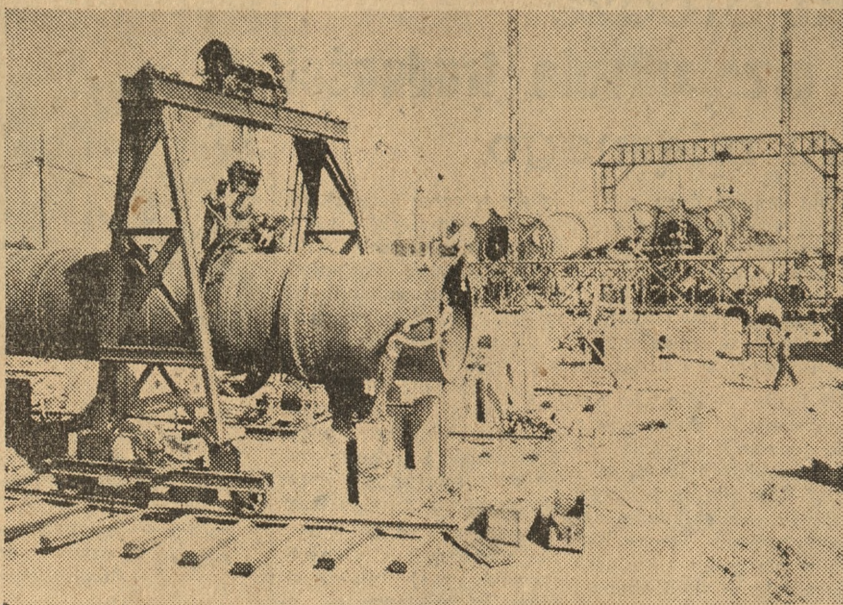
Budowa największej w Polsce cementowni w Wierzbicy postępuje szybko naprzód. W rekordowym tempie jedenastu dni zmontowano dwa największe piece obrotowe do wypalania cementu. Przy montażu zastosowano system inż. Cezarego Lubieńskiego, laureata tegorocznej nagrody państwowej. Na zdjęciu: Ogólny widok budowy. Na pierwszym planie brygada Henryka Bie- guły wyrabiająca 125 procent normy, podczas montażu pieca obrotowego do suszenia miazgi węglowej.
