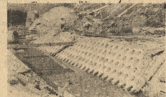
Fot. (3) K. Przychodzki Koryto odpływowe poza jazem. Brzegi wzmocniono pustobetonami, materiałem po raz pierwszy użytym przy tego rodzaju budowlach. Woda rozbijająca się o otwory w pustobetonach i kamienie wmurowane w dno — da charakterystyczny plask górskiego potoku.
