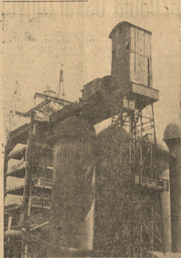
CAF fot. Banduch W dniu 21 lipca br. uruchomiona została w Odlewni „B” Zakładów Starachowickich pierwsza w Polsce potokowa linia formowania i składania odlewów. W tym samym dniu został po raz pierwszy zapalony nowy wielki piec. Potok w odlewni ruszył o 6 tygodni, a piec o 2 miesiące przed terminem.
