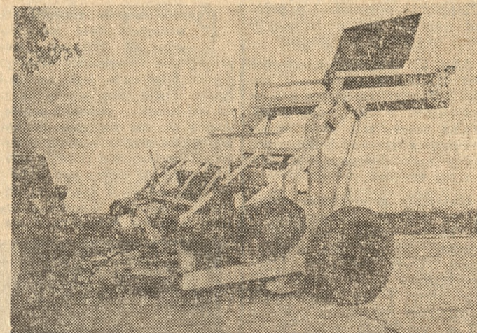
Na zdjęciu: prototyp MUK 1,7 kombajnu do zbierania kamieni. Fot. — Archiwum
