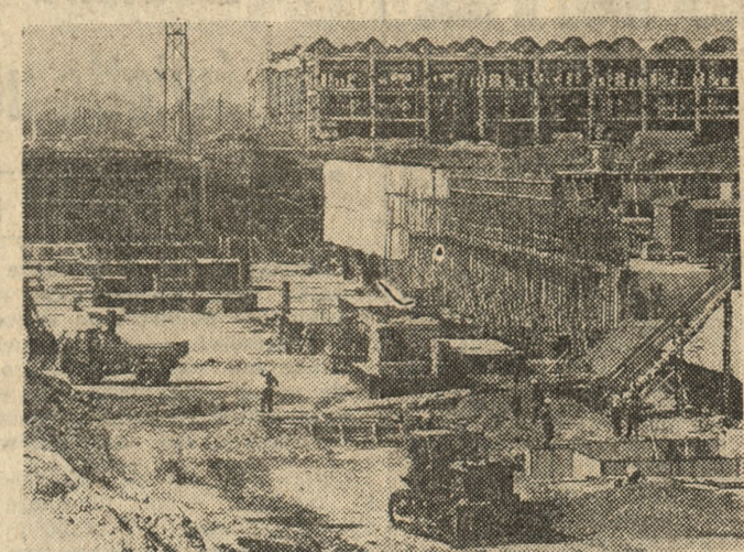
Na budowie elektrowni „Połaniec” stoją już fragmenty pod pierwszy kocioł, trwają prace przy wznoszeniu fundamentów budynku głównego, elektrofiltrów i kotła nr 2. Na zdjęciu: fragmenty wielkiej budowy.
