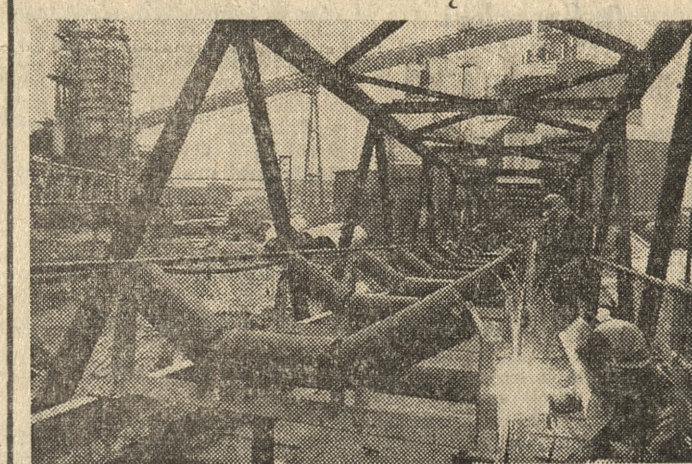
Przy realizacji Huty „Kałowice” wykonuje się obecnie roboty na ponad 900 obiektach. Na zdjęciu: montaż przenośnika.
