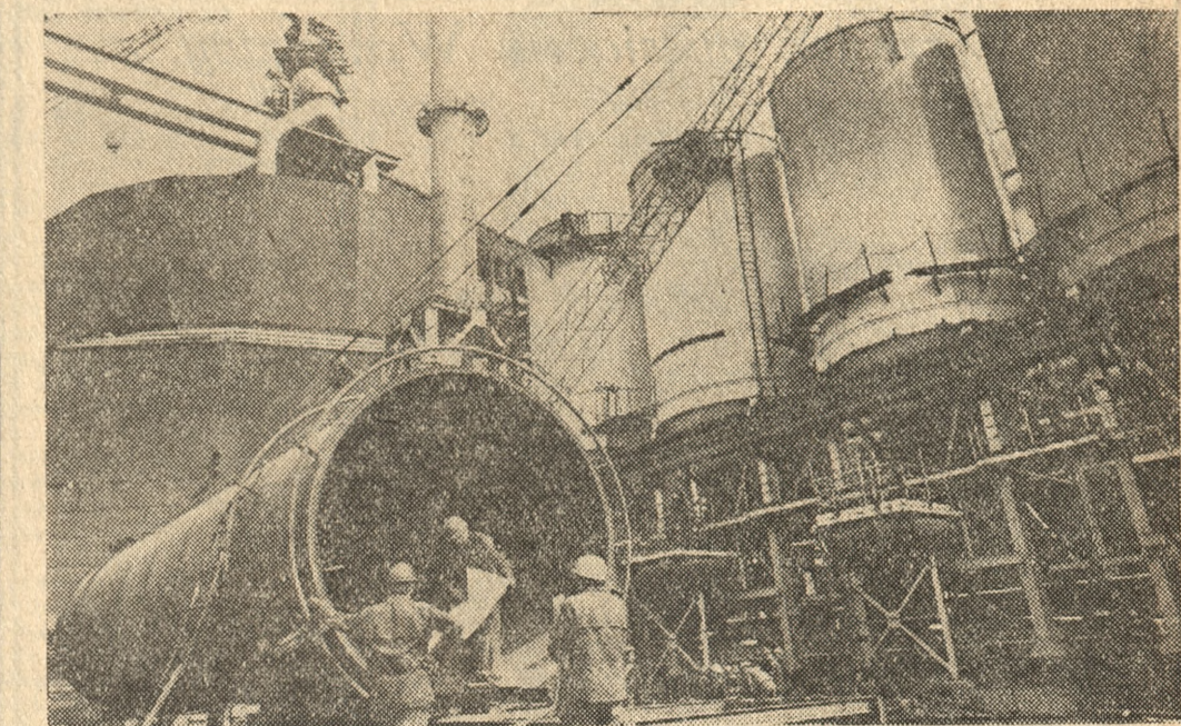
W szybkim tempie posuwają się prace przy budowie walcowni Huty „Katowice”. Fot. (2) — CAF
