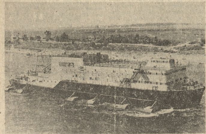
Pływające elektrownie „Zorza Polarna”, są niezasłapione na Dalekiej Północy, w pobliżu nowo odkrytych złóż surowcowych. Stacja — elektrownia ma specjalną instalację, która zapobiega wmarzaniu kadłuba w lód.
