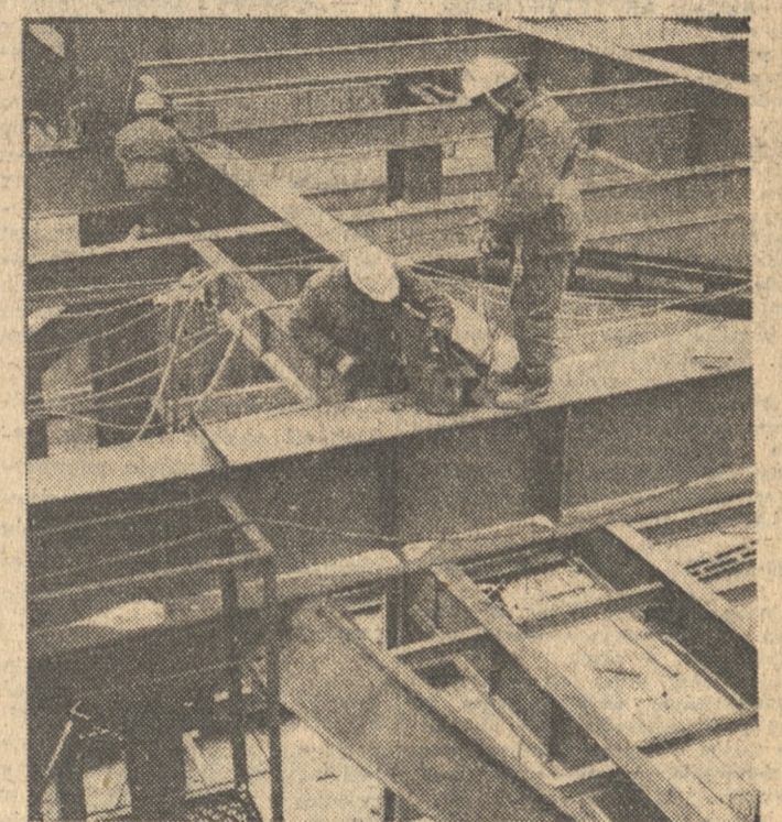
Trwa trzeci etap budowy elektrowni w Kozienicach. Mimo śniegu, wiatru i mrozu „ludzie ptaki” z warszawskiego Energomontażu — północ, zawieszani na linach montują stałą konstrukcję budynku kotłowni.
