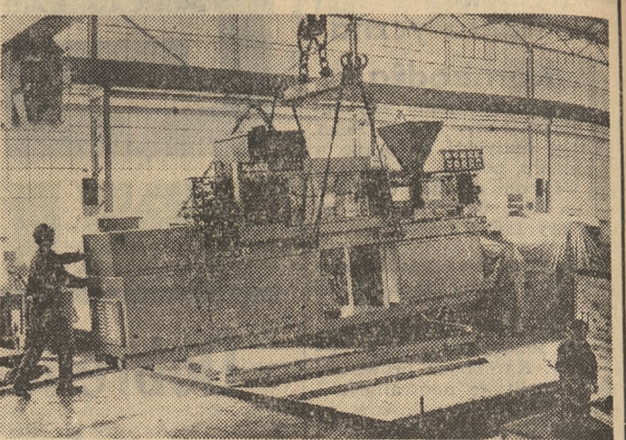
W ramach specjalizacji i kooperacji gospodarczej krajów RWPG zakłady w Freital (NRD) produkują wysokiej jakości automatycz- ne wtryskarki do mas plastycznych dla przemysłu chemicznego. Fot. — CAF
