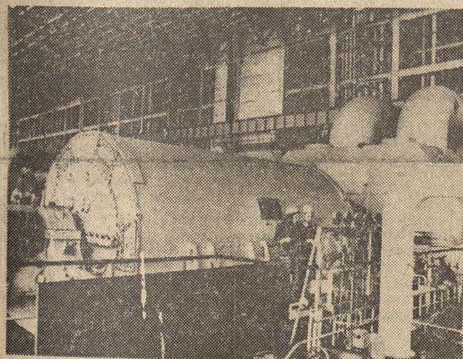
Największa w NRD elektrownia w Boxberg (na zdjęciu) o mocy 2 520 MW produkuje 20 proc. energii elektrycznej w tym kraju. Fot. — CAF
