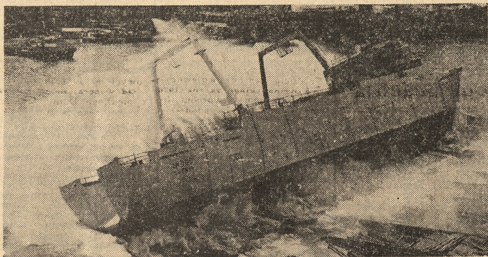
Siocznia Gdańska im. Lenina powiększa swój dorobek produkcyjny. 10 lipca zwodowano kadłub trawlera-przetwórnicy mł. „Indus”. Dopelnil on czteromilionową tonę nośności statków zwodowanych w okresie powojennym w tej siocznli.
