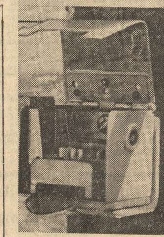
Ta mała skrzynka (zdjęcie górne) to nowy kasownik którym po służyć się będziemy od 1 lipca przy uniawianiu przejazdu. Na zdjęciu dolnym kasownik po otwarciu. Widoczne są małe bolce które po dowoim przesunięciu dają inny rozstaw dziurek. Pozwoli to na uniknięcie ewentualnych nieporozumień w wypadku kontroli. (za) Fot. (2) — H. Kamza
