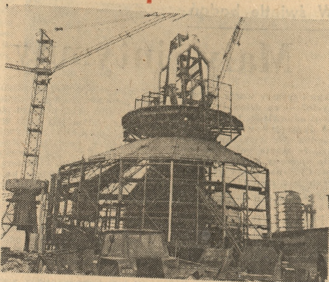
Tak wygląda konstrukcja przyszłego wielkiego pieca. Trzeba wierzyć autorowi tego zdjęcia, że na dachu są ludzie — monterzy. Ale to tak daleko, tak wysoko, że na fotografii nie sposób ich zauważyć.
