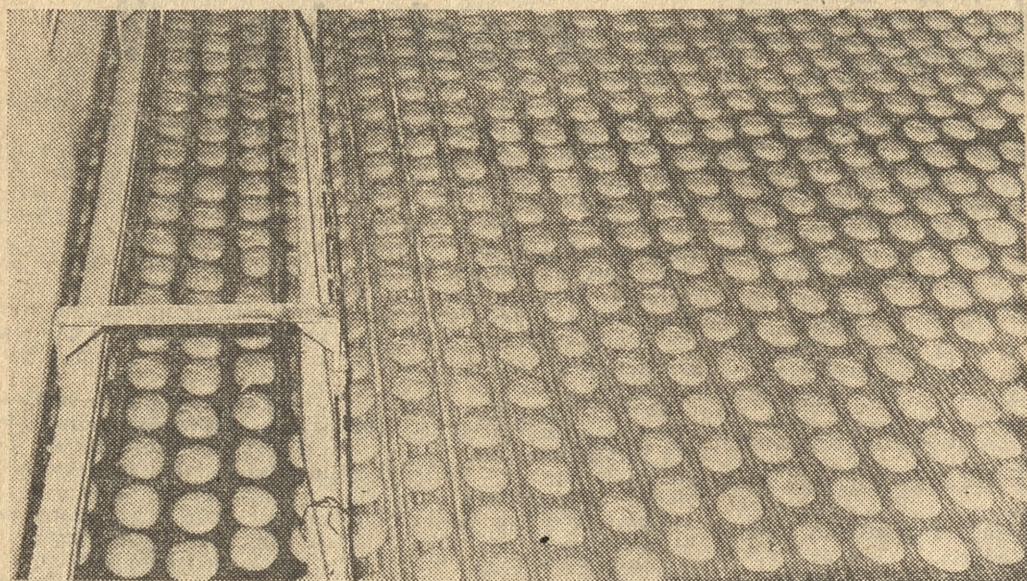
Piekarnia nr 5 przy ul. Żeromskiego w Poznaniu posiada najbardziej w grodzie Przemysław zmechanizowaną i automatyzowaną linię do wypieku bułek, która wyprodukowana została przez bydgoski „Spomasz”. Obsługuje ją zaledwie 5 osób, a w ciągu godziny wypieka się około 14 000 smacznych bułek (w dwóch rodzajach).
