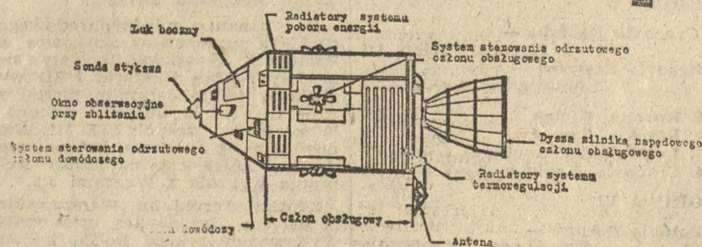
Człon dowódczy i obsługowy statku „Apollo” /JSM/
