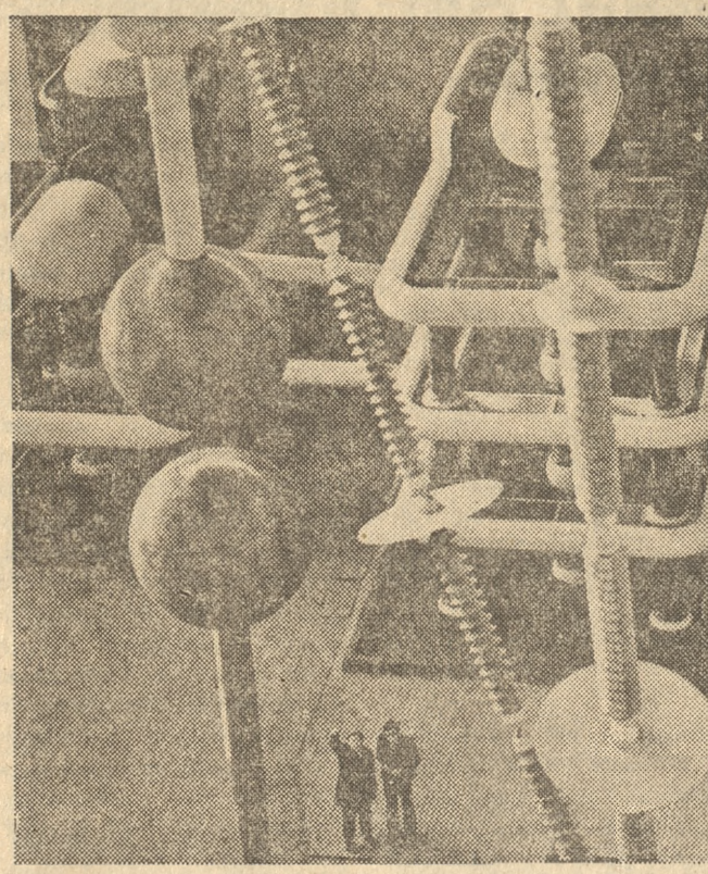
Laboratorium wysokich napięć
