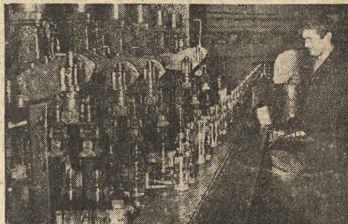
Na zdjęciu: automatyczna linia do produkcji butelek. Fot. — E. Kitzmann
