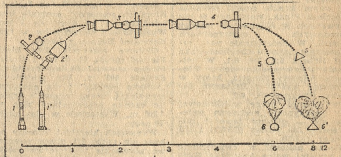
GRAFIK LOTU „SOJUZA” I „APOLLO”: (Czas w dobach od startu „Sojuza”) 1 — start „Sojuza”; 2 — wprowadzenie „Sojuza” na orbitę; 1' — start „Apollo”; 2' — wprowadzenie „Apollo” na orbitę; 3 — połączenie statków na orbicie; 4 — rozdzielenie statków; 5 — wejście „Sojuza” w atmosferę; 5' — wejście „Apollo” w atmosferę; 6 — lądowanie „Sojuza”; 6' — wodowanie „Apollo”.
