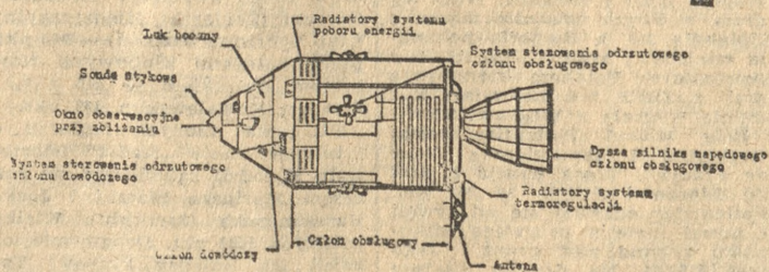
Całkowity dowódczy i obsługujący człony „Apollo” (PAI)
