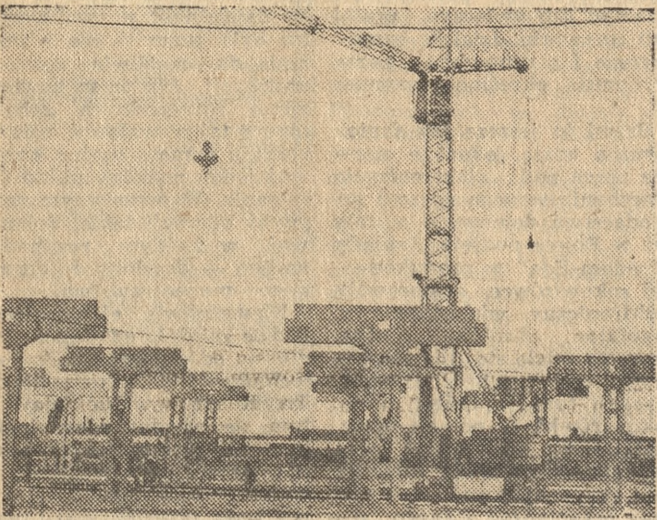
Słupy konstrukcyjne stwarzają już zarys przyszłej hali. Fot. — H. Kamza
