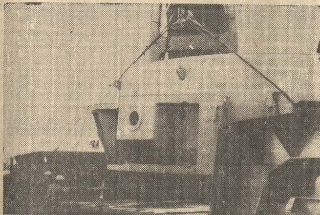
W porcie kolejowym Żurawica — Medyka przeładowano 3 bm. dwusety w br. wagon radzieckich urządzeń dla huty „Katowice”. Na zdjęciu: przeładunek 40-tonowego korpusu konwertora z radzieckiego wagonu — na polski.
