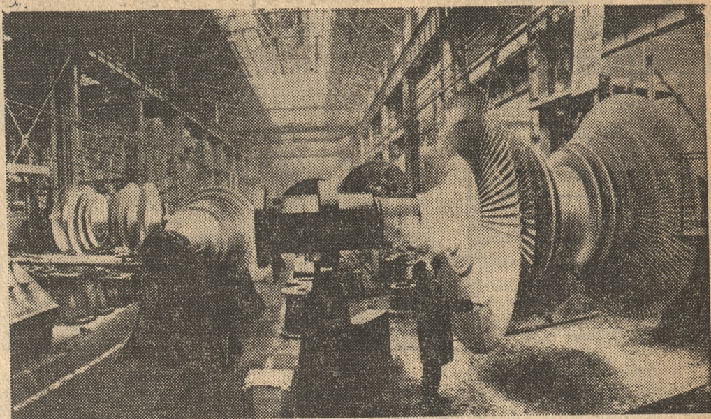
Wnętrze jednej z hal Zakładów Metalurgicznych im. XXII Zjazdu KPZR w Leningradzie. Dostarczają one krajom — członkom RWPG turbiny dla energetyki. Leningradzkie turbiny otrzymuje także energetyka polska.
