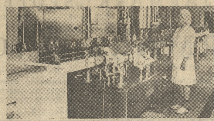
Na zdjęciu: fragment linii rozlewniczej nowych urządzeń. Fot. — H. Kamza
