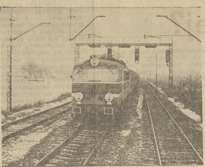
Elektrowóz EU-07, produkowany we wrocławskim „Pafawagu”, może prowadzić pociągi pospieszne z maksymalną szybkością 125 km/godz. PKP potrzebują mocniejszej i szybszej lokomotywy. Fot. — T. Talarczyk
