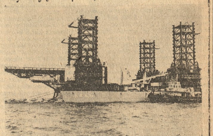
Pływającą platformę wiertniczą, zbudowaną przez stocznio- wów z Astrachania przewieziono do Baku. Po zamontowaniu u- rządzenie wierceń będzie szyby głębokości 6 km. CAF — TASS
