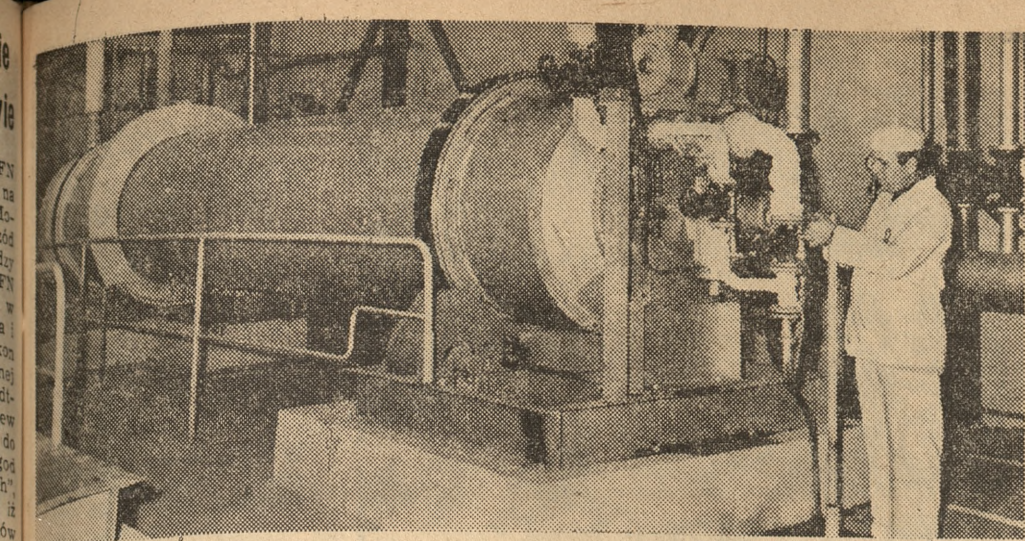
W Stawie pow. Słupca znajduje się jedna z najnowocześniejszych w świecie dekstryniarni. Wybudowano ją w rekordowym tempie — 15 miesięcy. Pierwsze tony dekstryny poszukiwanej m. in. przez przemysł włókienniczy, papierniczy a nawet wiertnictwo, opuściły zakład w Stawie jesienią ubiegłego roku. Na zdjęciu: Technologia produkcji jest tak zautomatyzowana, że zadaniem nielicznej załogi jest tylko obserwacja jej przebiegu. Fot. — H. Kamza
