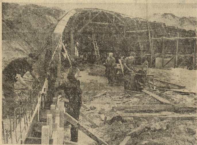
Na zdjęciu: pracownicy Poznańskiego Przedsiębiorstwa Budownictwa Przemysłowego nr 1 zatrudnieni przy budowie tunelu wjazdowego na stadion. Ma on być gotowy do 25 bm.
