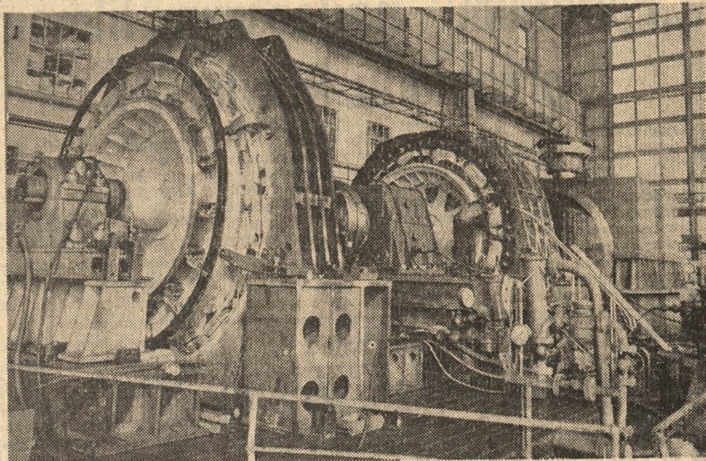
Wrocław. Dolnośląskie Zakłady Wytwarzające Maszyny Elektryczne opuszczają generatory o mocy do 200 megawatów. Widoczny na zdjęciu silnik otrzymany w Zawierciu. Dolnośląskie Zakłady współpracują także z poznańskim „Cegielskim” Fot. — H. Kamza
