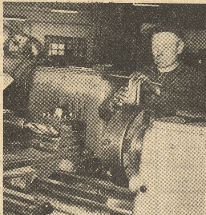
Tokarz Zygmunta Zajęca przy obróbce sprzęgła — urządzenia nieodzownego dla sprawnego działania oczyszczalni.
