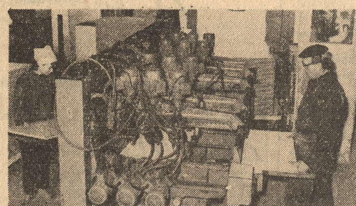
Wielowrzecionowa maszyna do wiercenia otworów. Jej zaletą jest możliwość wiercenia równocześnie 22 otworów przy operacji pionowej, a 10 przy operacji poziomej. Na zdjęciu: Daniela Kieres i Henryk Stróżyk przy obsłudze maszyny.
