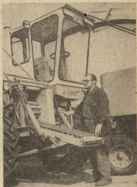
Sukcesem konstrukcyjnym jest samobieżny kombajn paszowy (wydajność 60 ton masy na godzinę). Załoga PFMŻ będzie musiała rozwinąć całą rodzinę podobnie nowoczesnych maszyn. Fot. — PIMR
