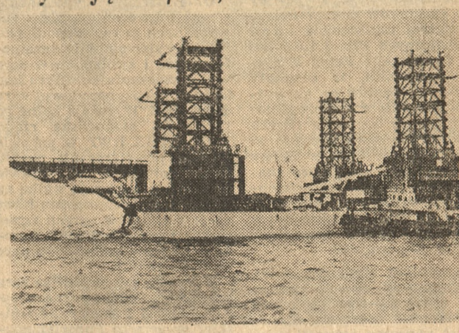
Pływającą platformę wiertniczą, zbudowaną przez stoczników z Astrachania przewieziono do Baku. Po zamontowaniu urządzenie wierceń będzie szyby głębokości 6 km.
