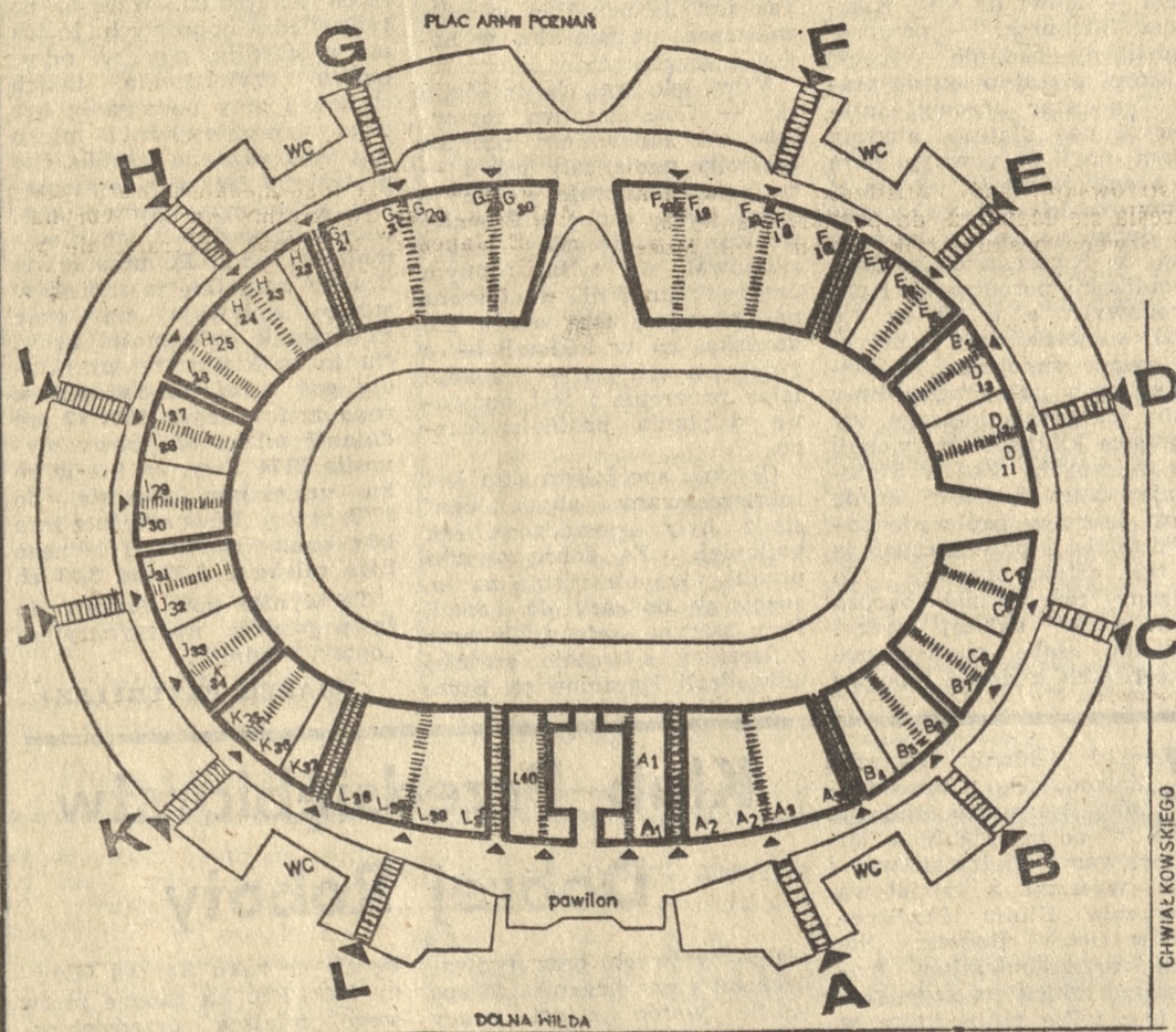
Schemat przebudowanego Stadionu im. 22 Lipca z zaznaczeniem sektorów i wejść.
