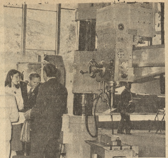
Wiertarka promieniowa 2M-55 do wiercenia otworów w tworzywie z różnych materiałów. Prezentuje ją na tegorocznych MTT w Poznaniu Związek Radziecki. Fot. — H. Kamza
