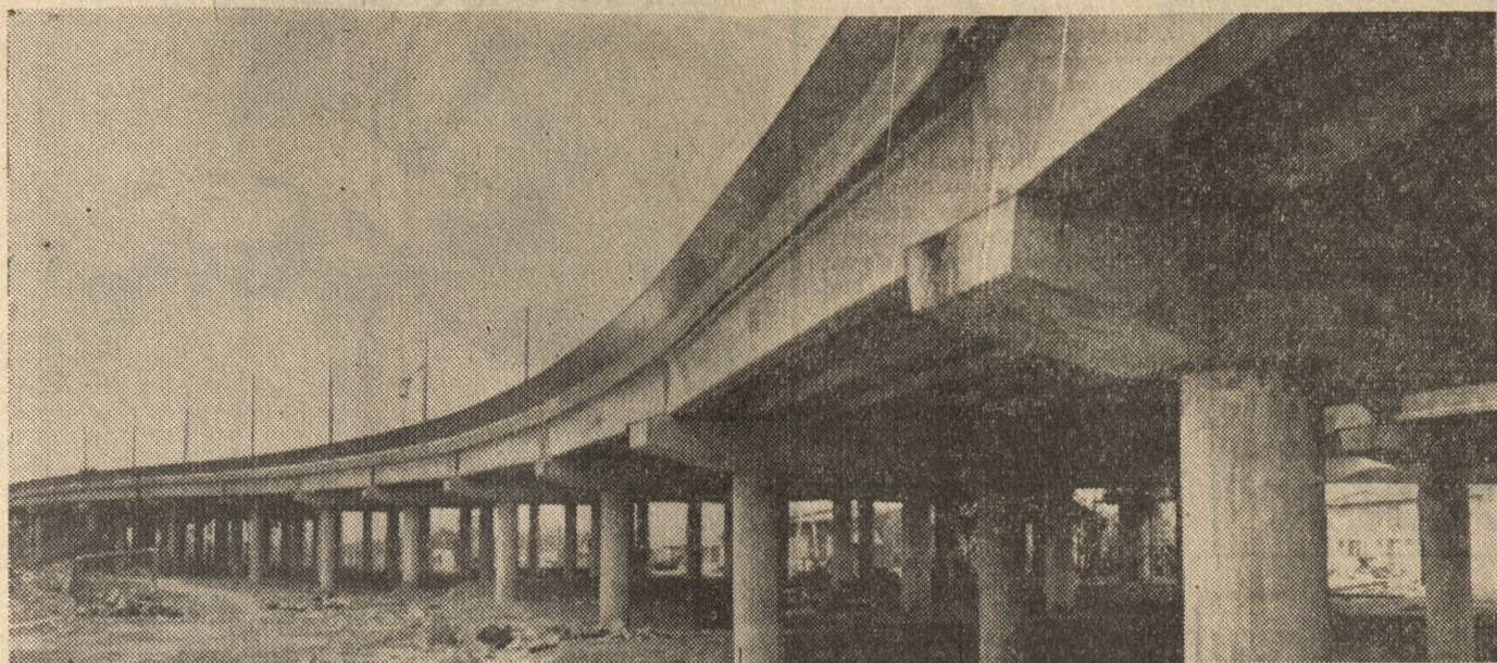
Trasa E-8. Nowoczesna wizytówka możliwości wielkopolskich robotników i inżynierów. W niespełna 18 miesięcy od wkroczenia na budowę pierwszych maszyn — do użytku oddany został odcinek Poznań — Września. Na zdjęciu: fragment wiaduktu.
