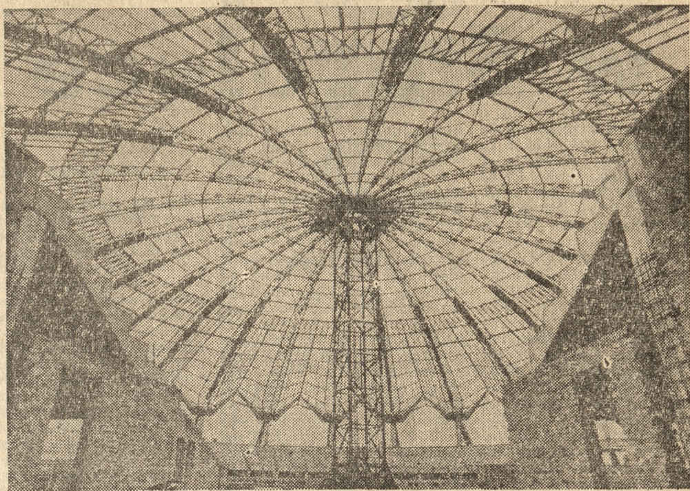
Tak, ale stalowa, bowiem jest to konstrukcja dachu nad halą widowiskowo-sportową przy ul. Jarochowskiego w Poznaniu.
