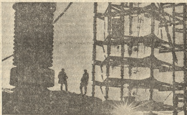
Generator udarowy widoczny na zdjęciu znajduje się w wysokogórskiej stacji badawczej „Anzob” w Tadżykistanie. Uczniowie badają tutaj wytrzymałość izolacji elektrycznej w warunkach wysokogórskich, dla potrzeb linii przesyłowych energii elektrycznej.
