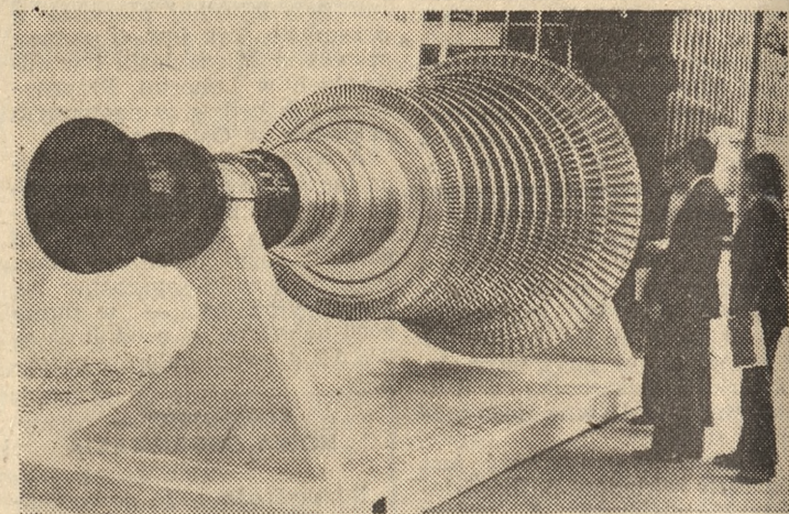
Wirnik turbiny o mocy 200 MW. Fot. — H. Kamza
