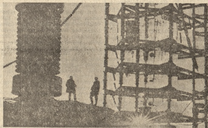
Generator udarowy widoczny na zdjęciu znajduje się w wysokogórskiej stacji badawczej „Anzob” w Tadżykistanie. Uczeń bada tutaj wytrzymałość izolacji elektrycznej w warunkach wysokogórskich, dla potrzeb linii przesyłowych energii elektrycznej.
