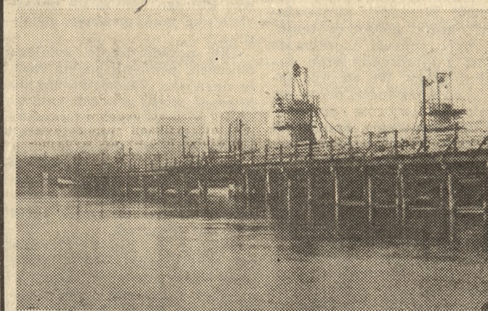
Trwają prace przygotowawcze do stawiania przęsła Mostu Łazienkowskiego w Warszawie. Na razie przez Wisłę została przerzucona kładka, z której korzystają robotnicy pracujący w kesonach.
