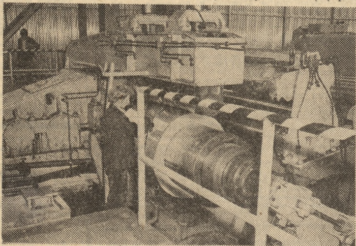
Zwizjarka — urządzenie rolujące rozwalcowaną blachę. Fot. — K. Przychodzki
