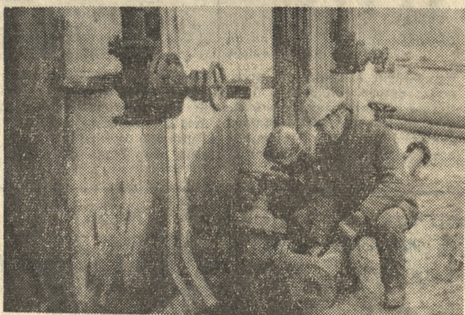
Na wyspie Wolin ekipy Przedsiębiorstwa Poszukiwań Naftowych z Piły prowadzą intensywne poszukiwania ropy naftowej. Na zdjęciu: brygada z PPN przy pracach montażowych na wiertni. Piotr Szerszeń (z prawej) i Zbigniew Maciaszczyk instalują przewody rurowicowe przy zbiornikach.
