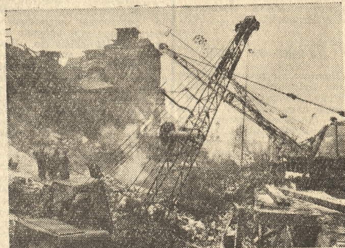
Olbrzymimi dźwigami usuwa się poszczególne elementy zwaliska gruzu, które pozostało po kilkukondygnacyjnym budynku magazynu „Stomila“.
