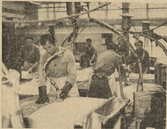
Modernizacja Gnieźnieńskich Zakładów Garbarskich objęła również procesy technologiczne garbowania skór. Jedną z nowości jest sirżenie skór przed garbowaniem.
