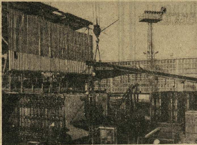
Fragment form bateryjnych do elementów ścianowych i stropowych.
