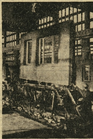
Gotowy element ściany ustawia się na specjalnym wózku, który następnie mała lokomotywa przewozi na miejsce budowy. CAF — fot. Staszyszyn
