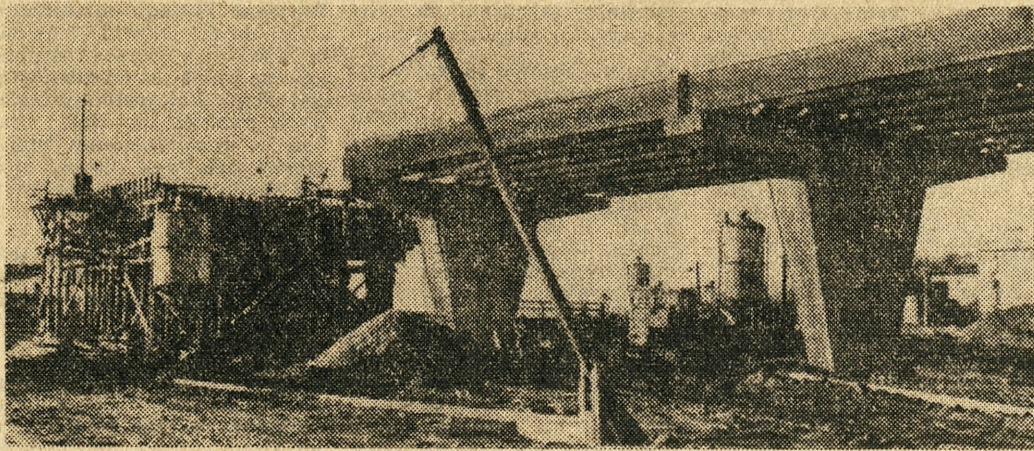
Najtrudniejszy etap budowy wiaduktu, to realizacja jego środkowych przęseł, która odbywa się podczas normalnego ruchu pociągów.
