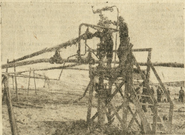
Płatanina rur, to kopalnia. Tak z zupełnie prozaicznie wygląda urządzenie do wydobywania siarki metodą podziemnego wytopu. Tym sposobem wydobywana jest 70 procent polskiej siarki. CAF — fot. Kwiatkowski
