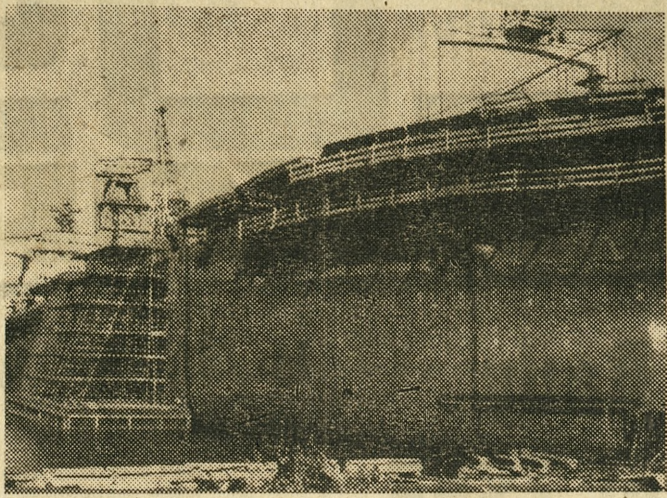
Pod koniec lipca największy statek zbudowany w polskich stocznich 55-tysięcznik m/s „Manifest Lipcowy” wypłynie w próbnym rejsie. Na zdjęciu: „Manifest Lipcowy” przy nabrzeżu wyposażenia w stoczni gdyńskiej im. „Komuny Paryskiej”. CAF — Uklejewski
