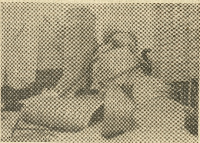
W Newton [USA] wybuch jednego z 36 silosów załadowanych ziarnem spowodował swoistą reakcję łańcuchową, wywracając blisko stojące następne silosy. W efekcie wysypało się ponad 25 tys. ton ziarna.
