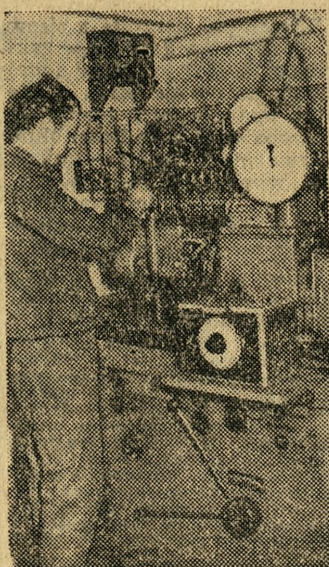
Jednym z nowoczesnych urządzeń pomocnych przy naprawie samochodów i ciągników PKS, jest sprowadzony z Austrii aparat do badania pomp wtryskowych. Na zdjęciu: pracownik warsztatowy L. Grześ sprawdza jedną z oddanych do naprawy pomp.
